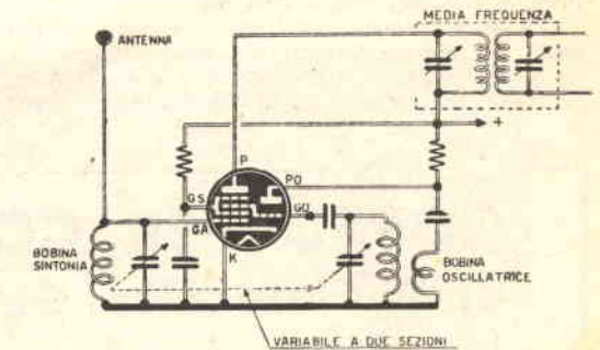
Fig. 4. - In pratica per la conversione di frequenza non si fa uso di una valvola come quella della fig. precedente, bensì di una valvola versione di frequenza mediante un triodo-esodo molto più complessa. Qui è rappresentata la con-
