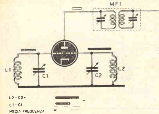
Fig. 3. - Qui sopra è sintetizzato un circuito cambia-frequenza, in cui C1 e L1 rappresentano il circuito di sintonia, C2 e L2 quello oscillatore, e MF1 la Media Frequenza.
